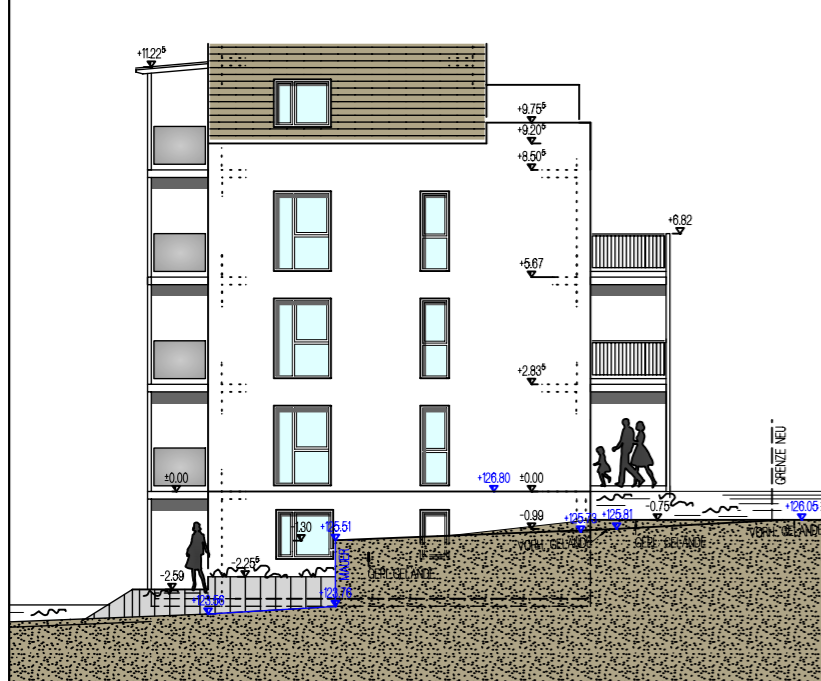
ANSICHT NORDEN
